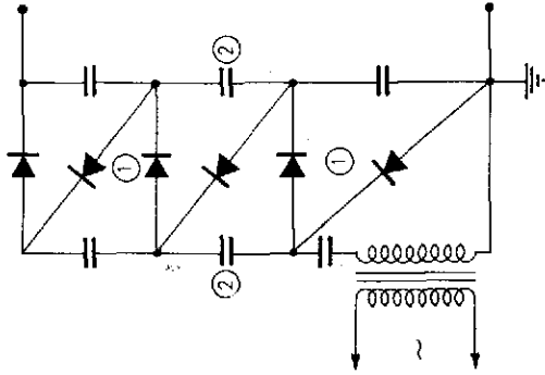
ACELERADOR DE COCKCROFT—WALTON
